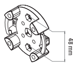
132303 Universallager TK48 verstärkt 50 Nm
