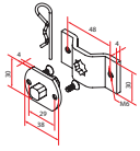
A3506_0552 Lager TK 60, mit 10 mm Innenvierkant
