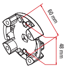
132300 Universallager TK48 u. 60 Vorbau bis 30 Nm
