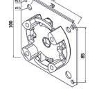
132323 Universallager auf Platte 100 x 100 mm bis 30 Nm (Kömmerling)
