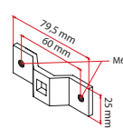
132328 Lager TK 60, mit 10 mm Innenvierkant
