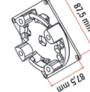
132329 BK-Lager bis 30 Nm
