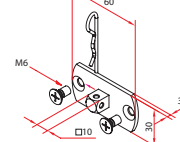
A4506_0580 Vierkant 10 mm mit Platte M6 Gewinde
